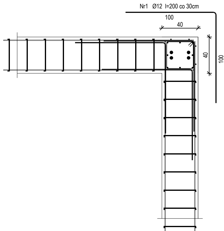
Wykaz zbrojenia
