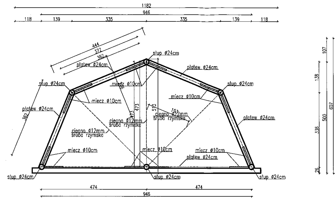
Rzut więźby
