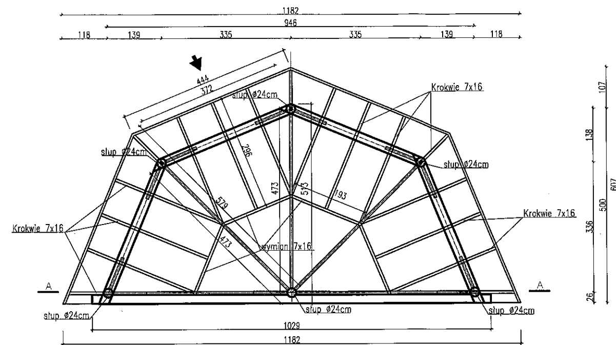
Rzut więźby
