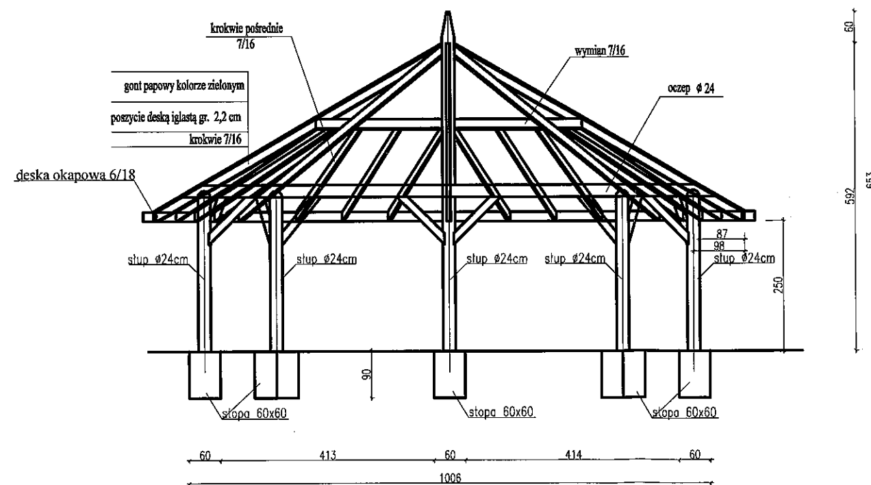
Przekrój A-A
