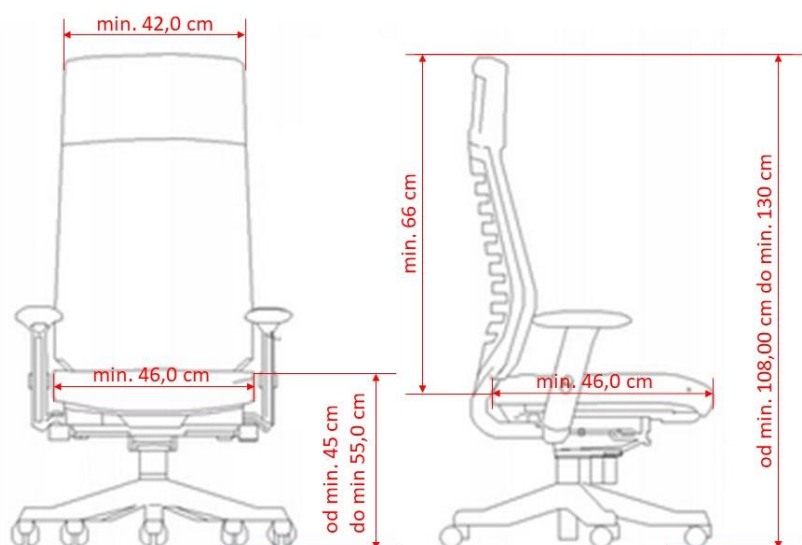
Rys. 1 Krzesło biurowe na kółkach - Rysunek poglądowy.
