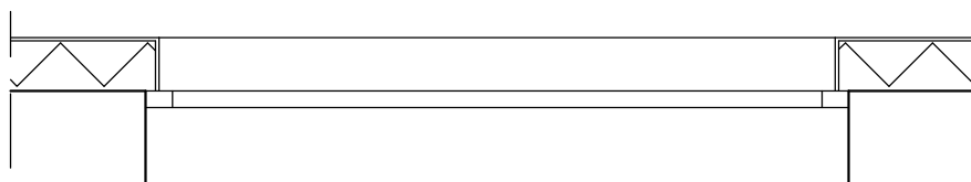
1B. rzut_ montaż okna w ścianie płn. / wsch.
