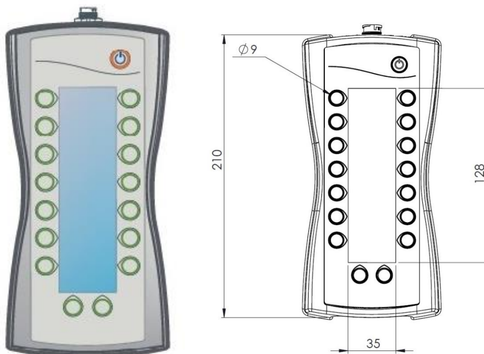
Rysunek schematyczny wymiary w mm
