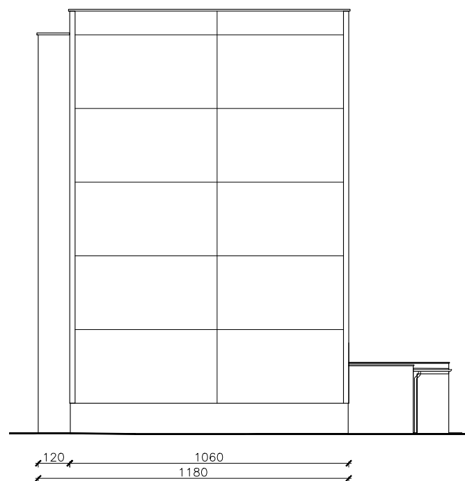
Elewacja wschodnia
