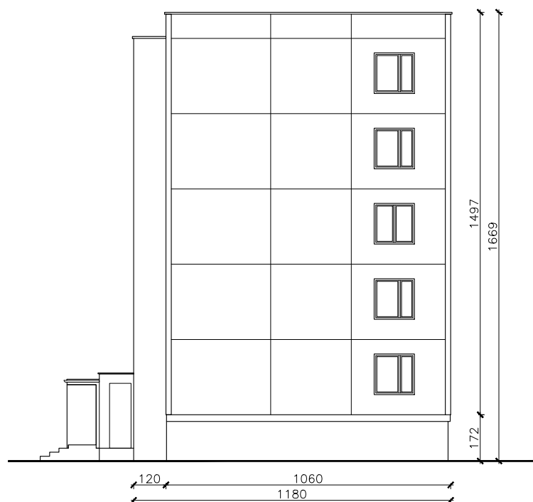
Elewacja wschodnia
