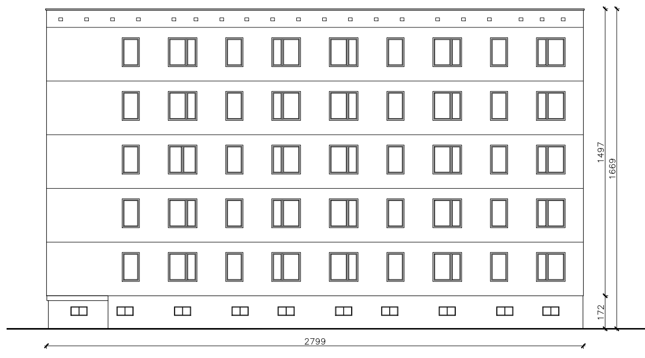
Elewacja północna
