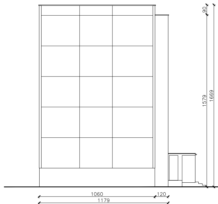
Elewacja zachodnia
