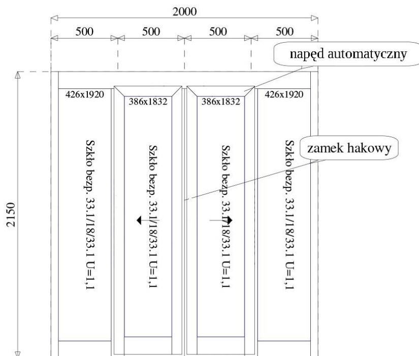
Rys. 1 Widok od strony zawiasów
