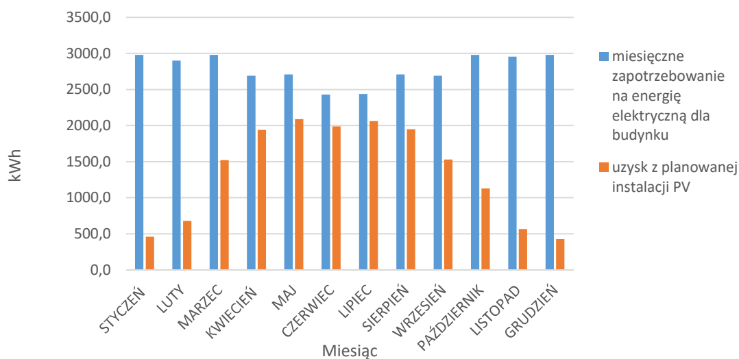
Bilans miesięczny zużycia energii elektrycznej wraz z miesięcznym uzyskiem z fotowoltaiki - Budynek "B" przy ul. gen. Pułaskiego 4/6
