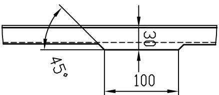
Szczegół C
