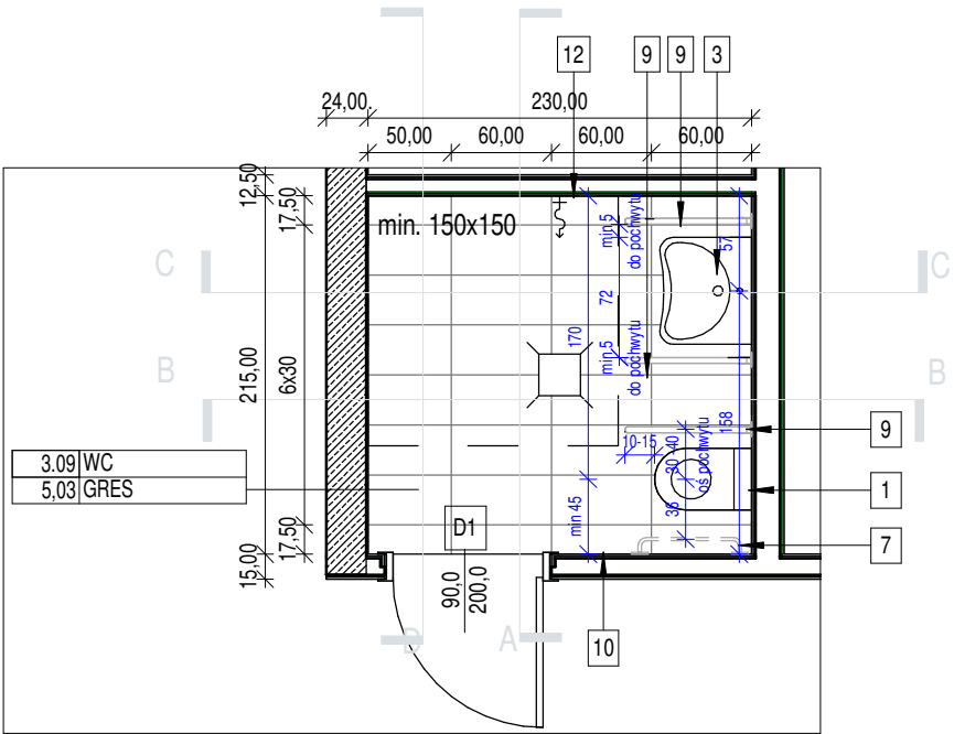
RZUT WC DLA OSÓB Z NIEPEŁNOSPRAWNOŚCIAMI 1 : 50
