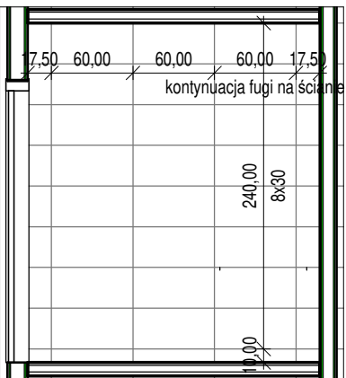
WIDOK D-D 1 : 50
