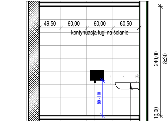
WIDOK C-C 1 : 50
