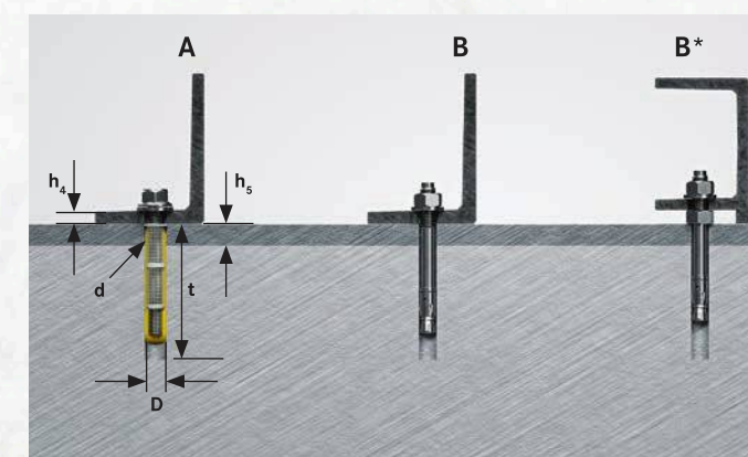
(A) Kotwa chemiczna (B) Kotwa mechaniczna
