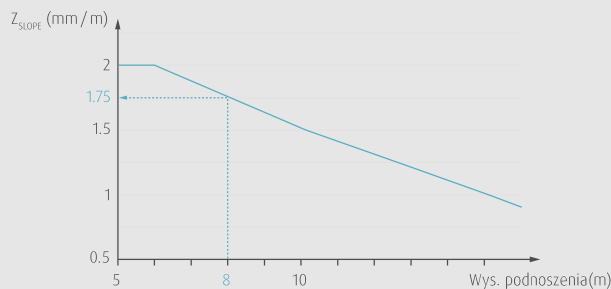
Rysunek 3 - Określenie Z_{\text{SLOPE}}
