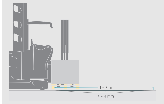
Rysunek 6 - wymiary wzdłuż korytarza
