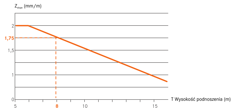
Rysunek 2: Określenie współczynnika Z_{slope}
