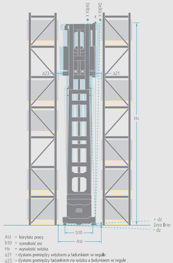
Rysunek 5 - Odchylenia boczne wózka
