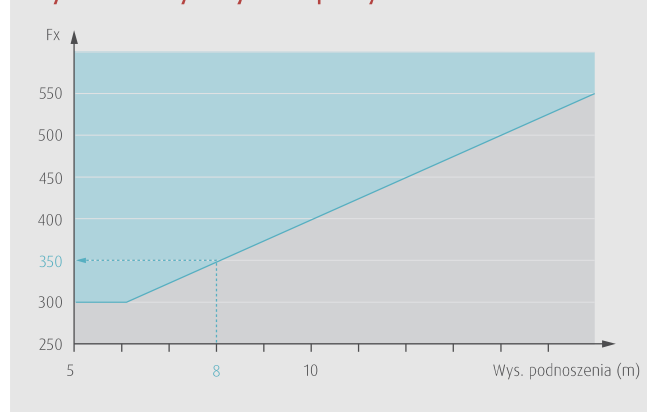
Rysunek 7 - Wymiary dla współczynnika zmienności Fx
