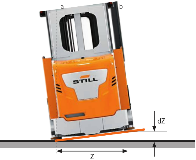
dZ = różnica wysokości; Z = rozstaw kół podporowych wózka; a, b = koła podporowe Rysunek 1. Poprzeczne różnice wysokości
