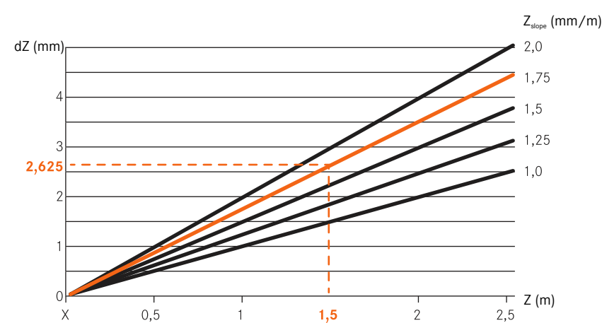
Rysunek 3: Obliczenie maksymalnej dopuszczalnej różnicy wysokości dZ
