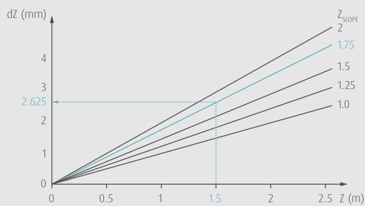
Rys. 4 - Obliczanie dZ
