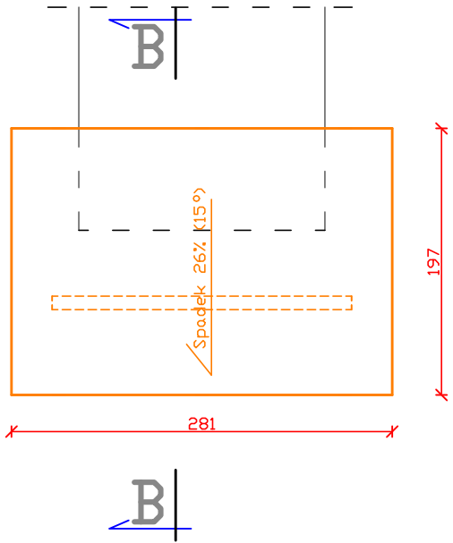
RZUT DACHU 1:50
