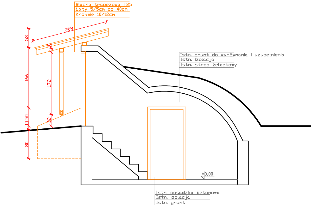
PRZEKRÓJ B-B 1:50
