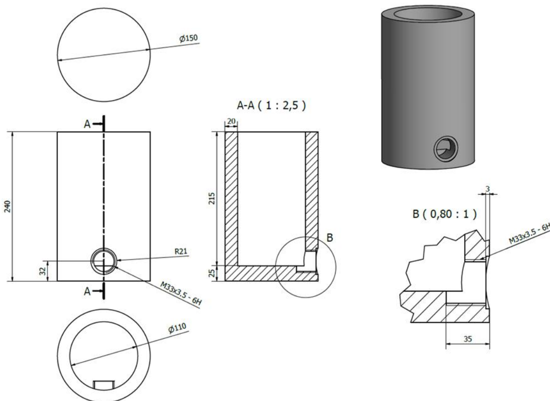
Rys.1. Specyfikacja Tygiel Φ150mm, materiał – grafit HLM
