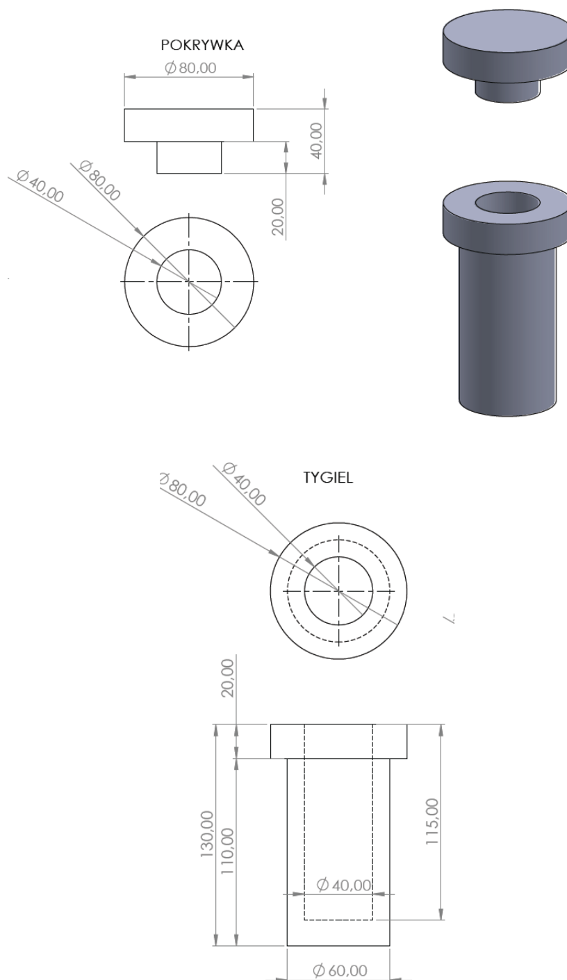
Rys.3. Specyfikacja tygla z pokrywką, materiał – grafit HLM, ilość 100 sztuk
