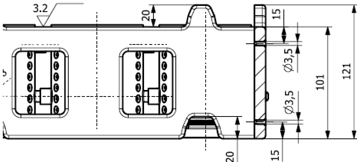
WIEKO (POKRYWA) FORMY SEROWARSKIEJ
