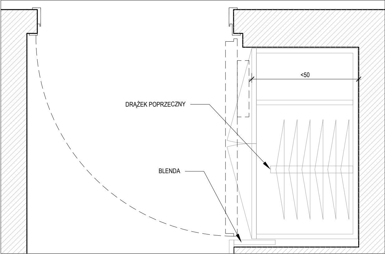
NIETYPOWY UKŁAD SZAFY - PRZYKŁAD 1 SKALA 1:10
