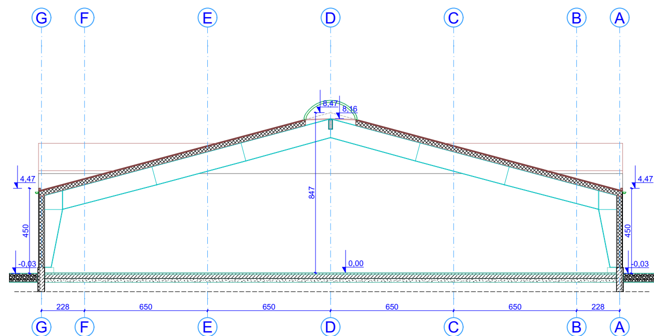
PRZEKRÓJ B-01
