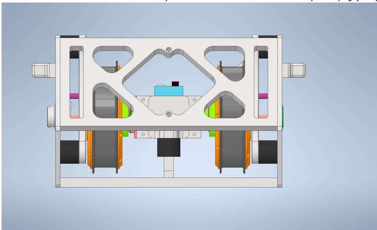
Rys.2 – Stanowisko do badań silników – widok z przodu
