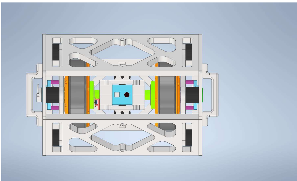
Rys.4 – Stanowisko do badań silników – widok z góry
