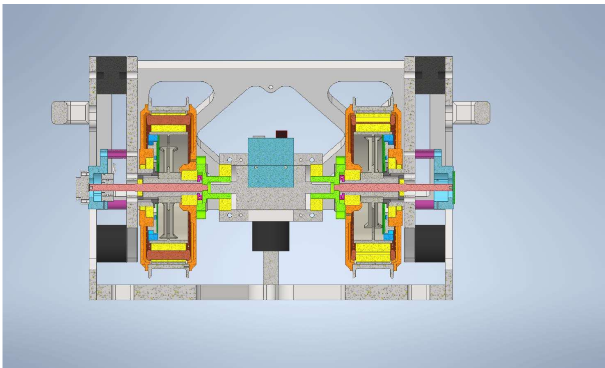
Rys.5 – Stanowisko do badań silników - przekrój
