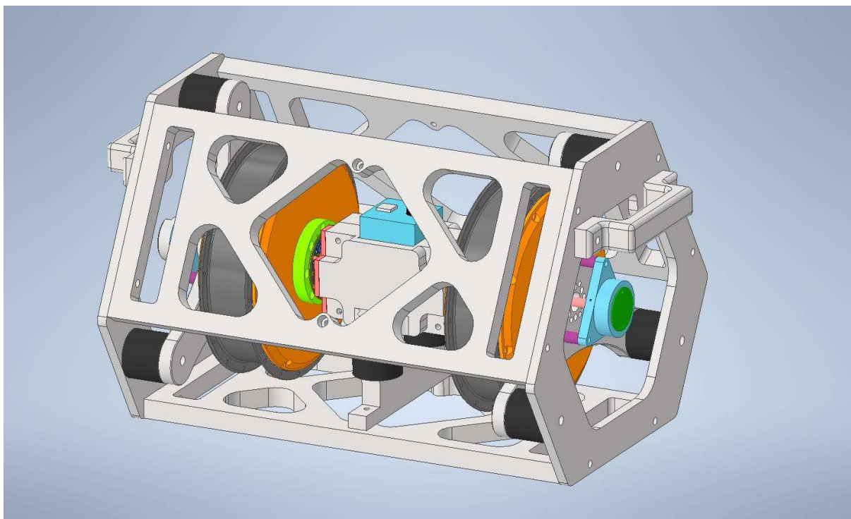
Rys.1 – Stanowisko do badań silników - rysunek poglądowy
