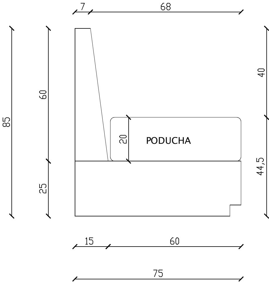
PRZEKRÓJ, WYMIARY NA GOTOWO (Z OKŁADZINAMI)
