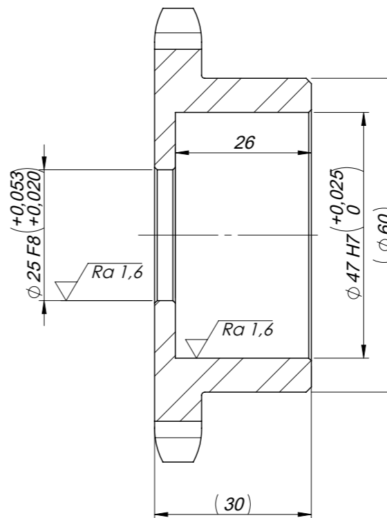
PRZEKRÓJ A-A
