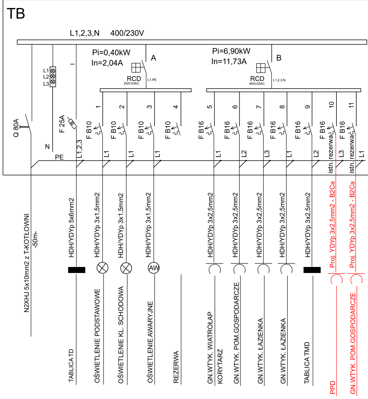
Rys. nr 2, schemat rozdzielnicy TB
