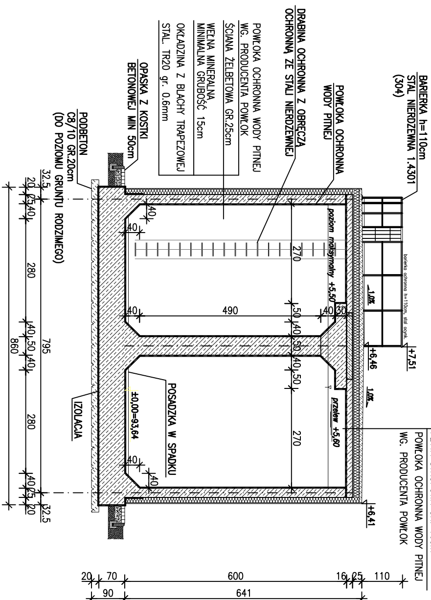
PRZEKRÓJ A-A
