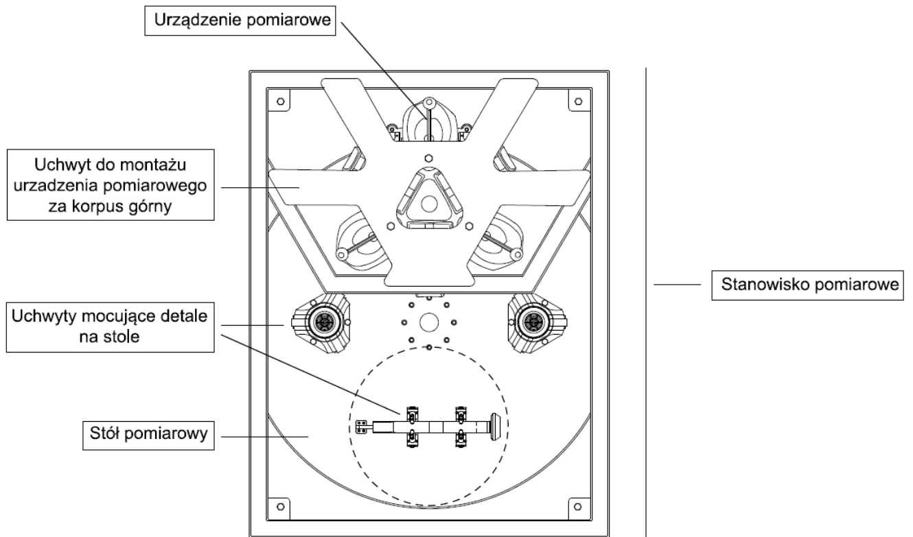
Rysunek ideowy celi pomiarowej.
