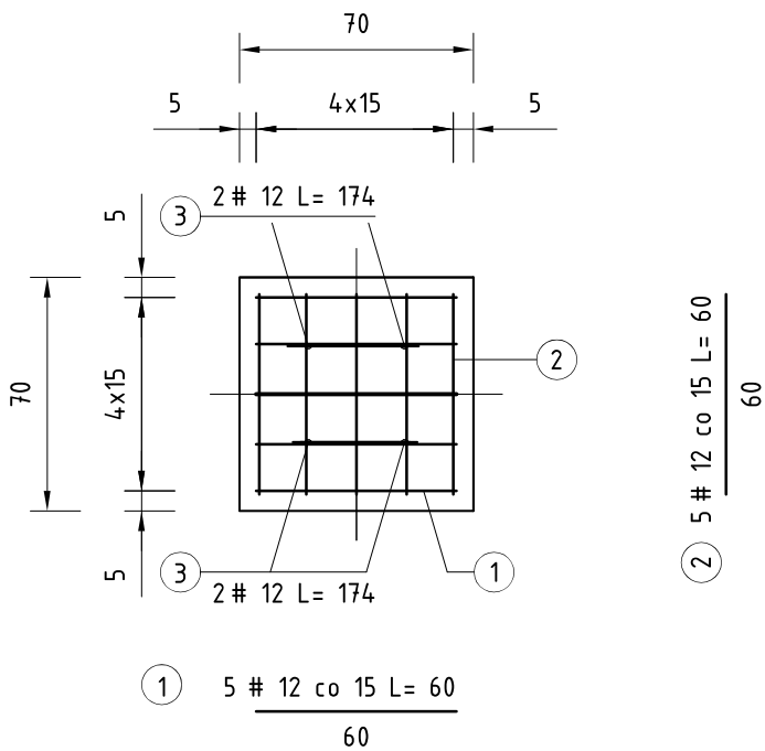
PRZEKRÓJ 1-1
