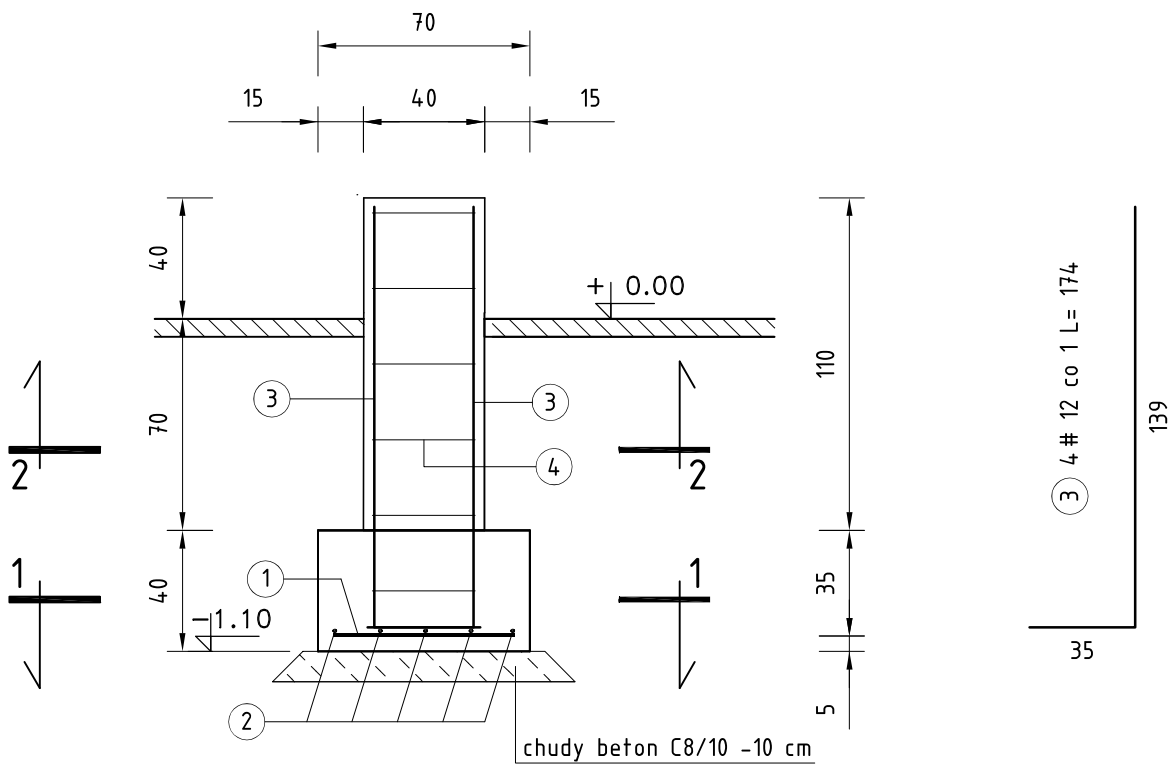
PRZEKRÓJ 2-2
