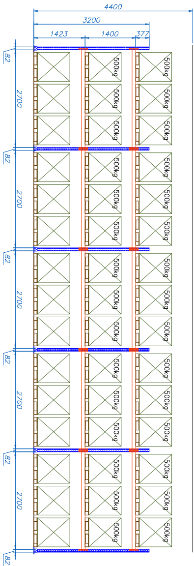
Regał paletowy
