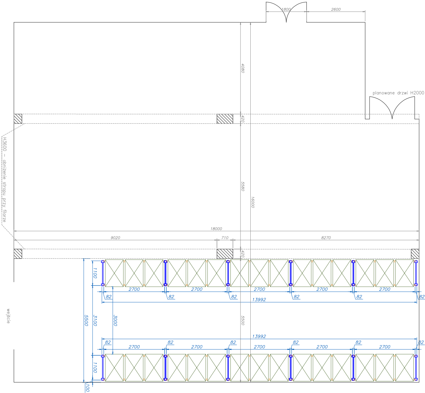
Regał paletowy
