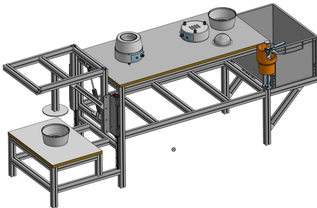
Rysunek poglądowy stołu roboczego
